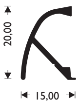
M 11116 ΝΕΡΟΧΥΤΗΣ W=184 gr/m DRIP
